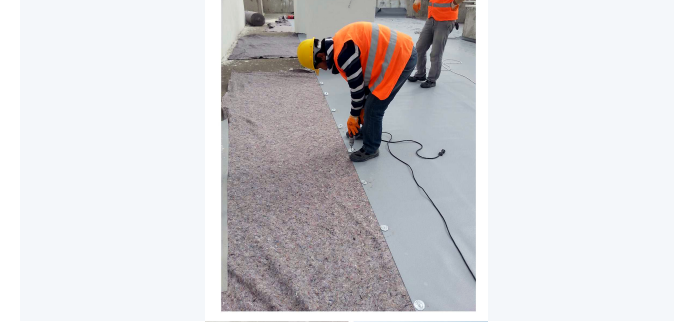
Uygulama detayı
