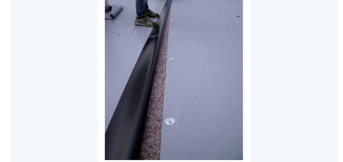
Birleşim detayı
